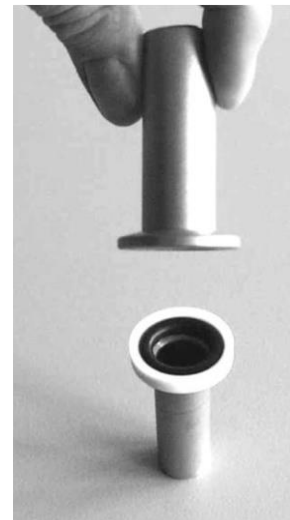
Abb. 53: Kleinflansch und Zentrierring mit Kleinflansch
