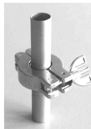
Abb. 55: Festziehen des Spannrings
