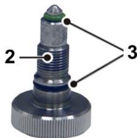
Abb. 56: Ventilöffnung und Ventileinsatz mit O-Ringen (Beispielabbildung, variiert je nach Anlagentyp)
